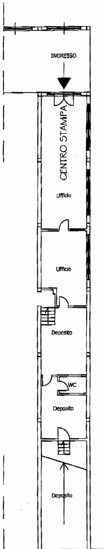
Pianta Centro Stampa "ex Officine" - Via P.E. Castagnola Scala 1:200
